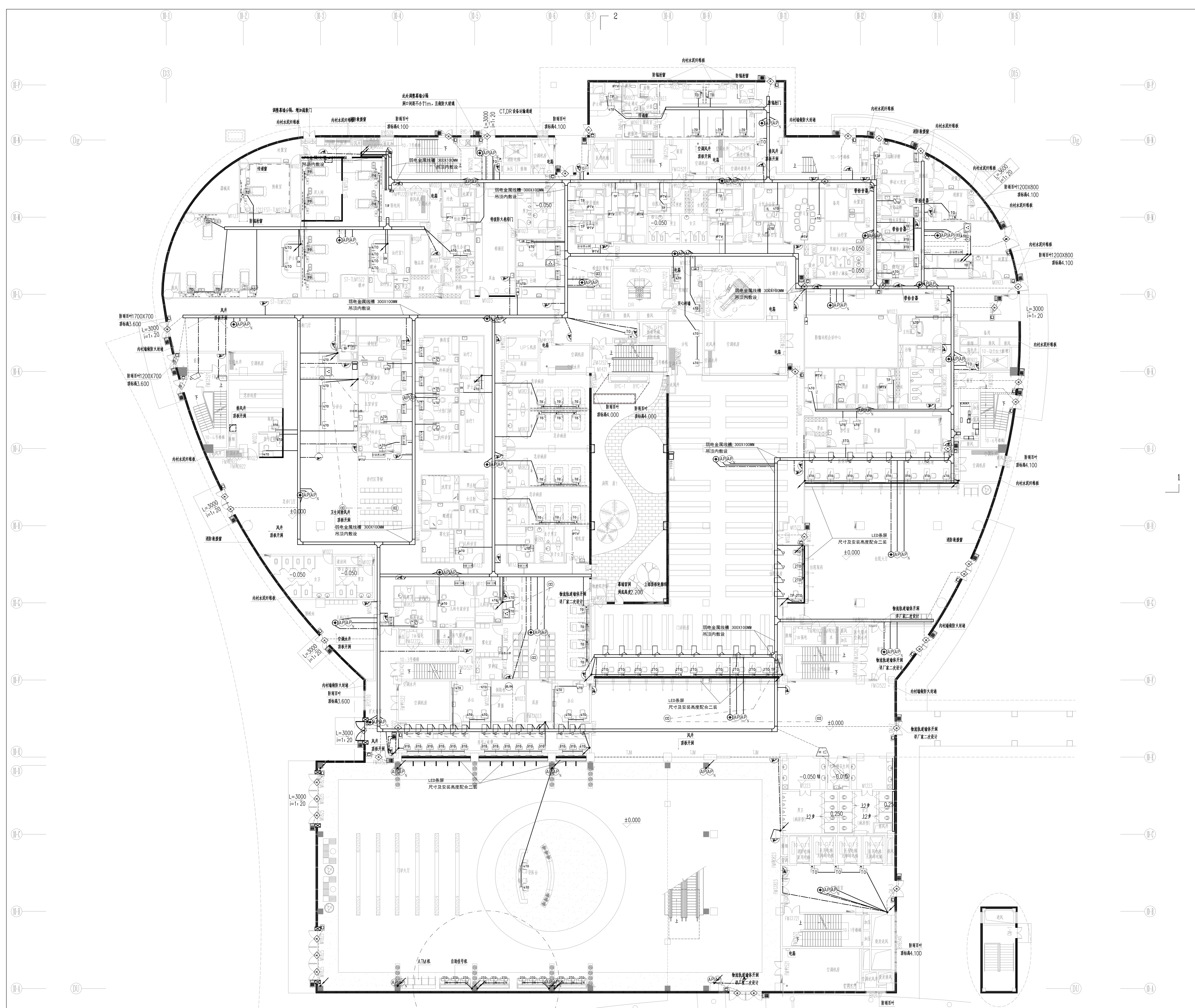
一层弱电平面图 (一) 1:150
